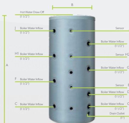
Dimensions (300-2000L)
