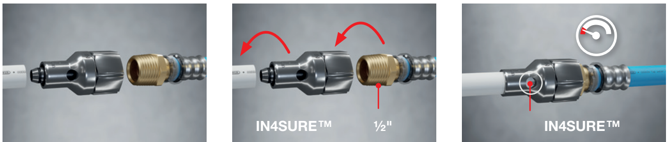
Fig. 29: Pressure check with coupler: 16 mm: 4013571 - 20 mm: 4013572 - 25 mm: 4013573.
